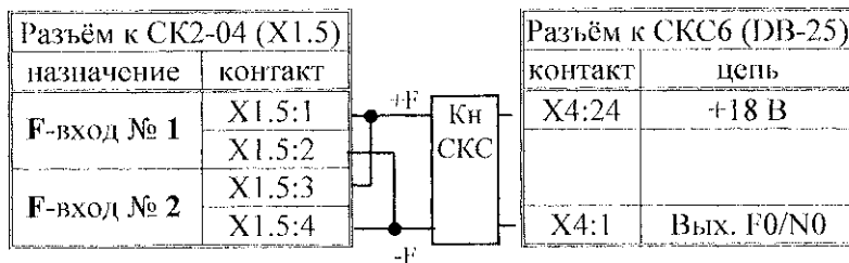
Рисунок Д.5 - Распайка разъемов к СКС6 и подключение к разъёмам СК2-04 для подключения частотных сигналов
