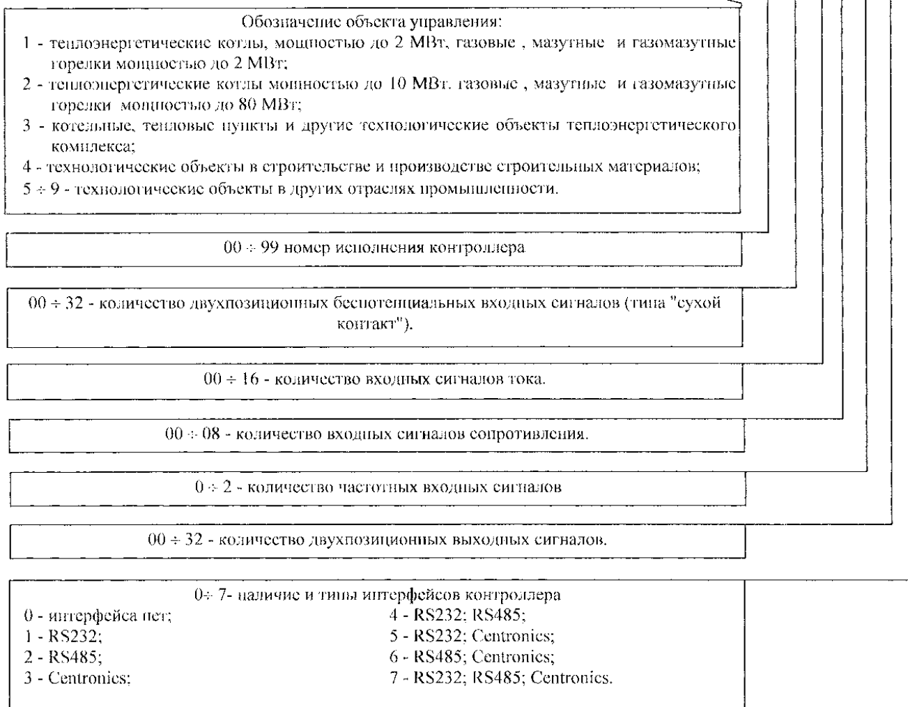
Рисунок 2.1 - Расшифровка условного обозначения контроллера На лицевой панели контроллеров нанесено:
