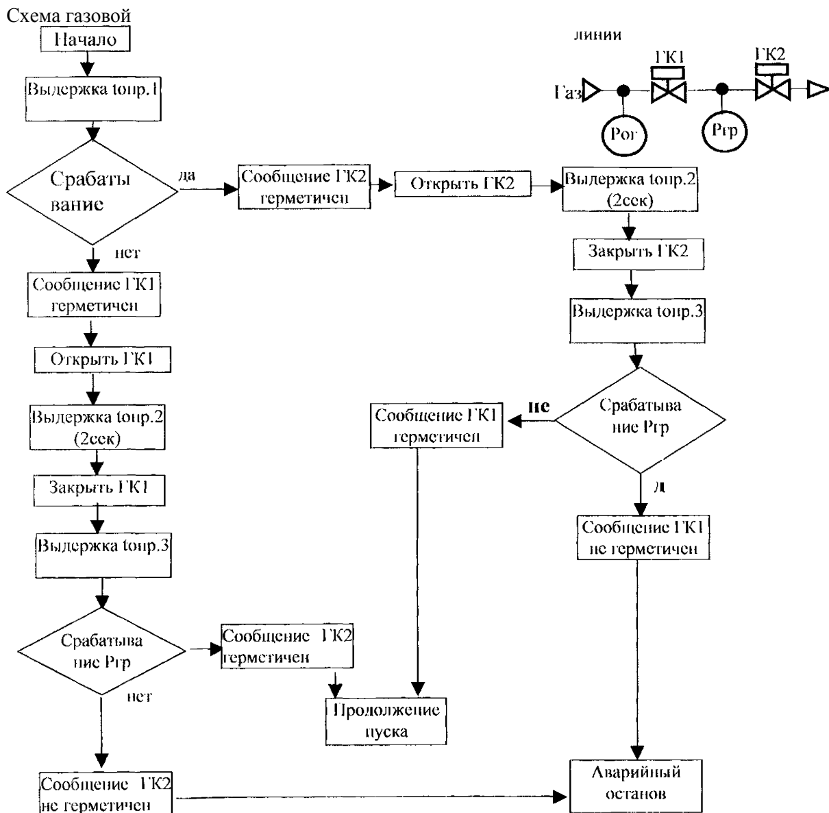
Рисунок Б.2 - Алгоритм проверки при наличии ГК1, ГК2, отсутствии ГКП ()
