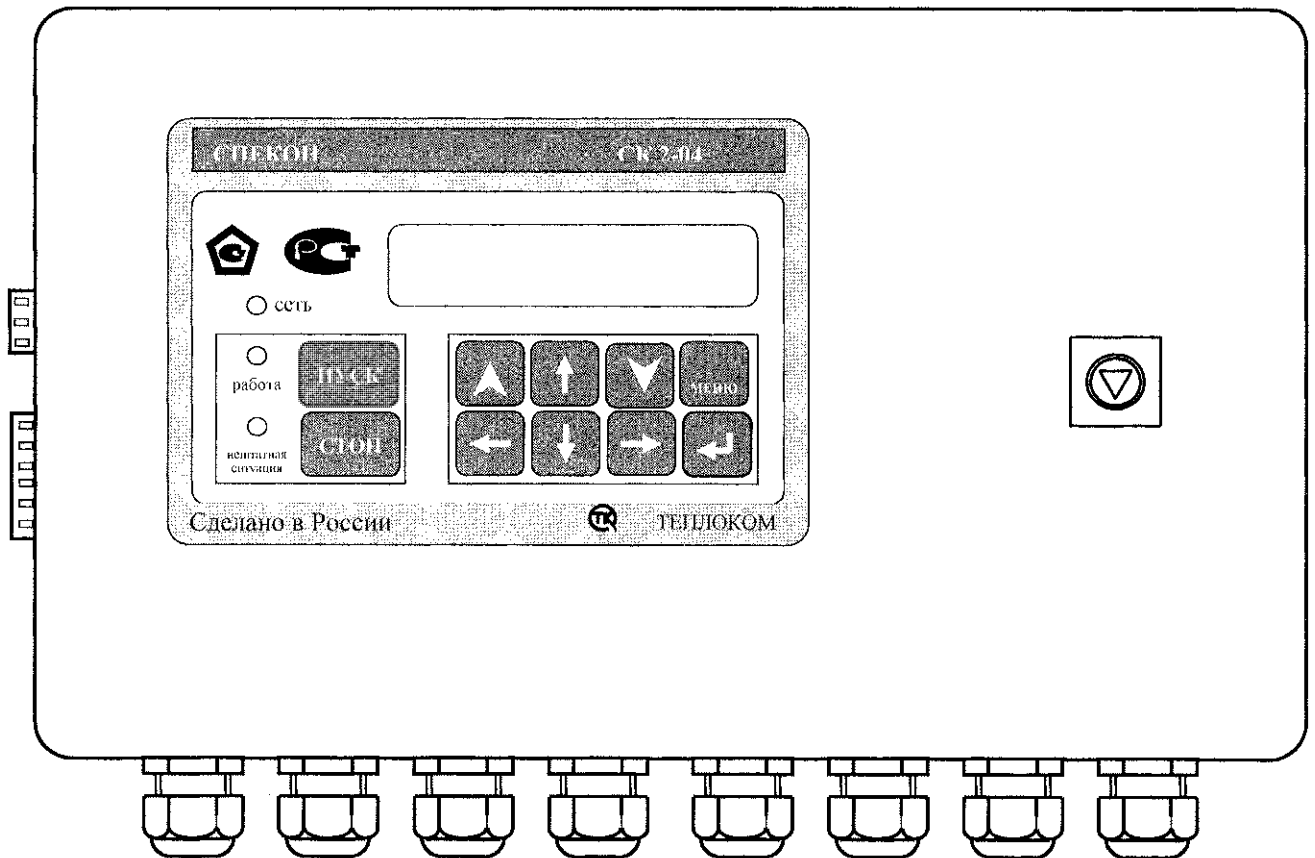
Рисунок 3.1 - Внешний вид контроллера (вид спереди).
