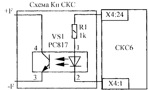
Рисунок Д.5 - Распайка разъемов к СКС6 и подключение к разъёмам СК2-04 для подключения частотных сигналов
