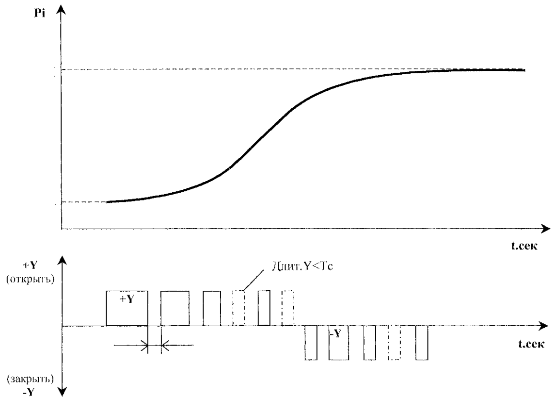
Рисунок В.3 - Оптимальная работа ПИД-регулятора
