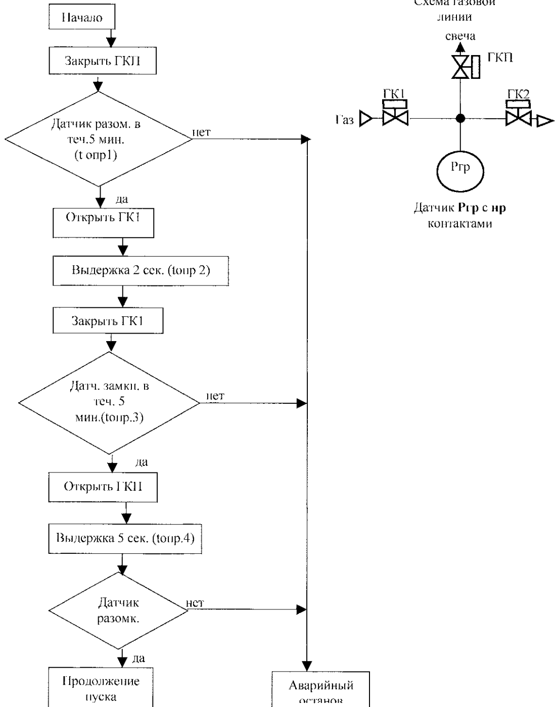
Рисунок Б.1 - Алгоритм проверки при наличии ГК1, GK2, GKП
