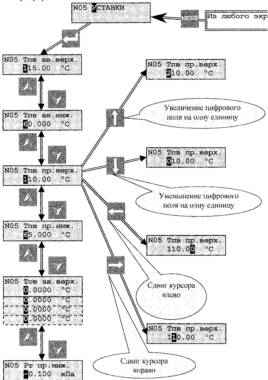
Рисунок 6.5 - Раздел меню наладчика «Уставки»
