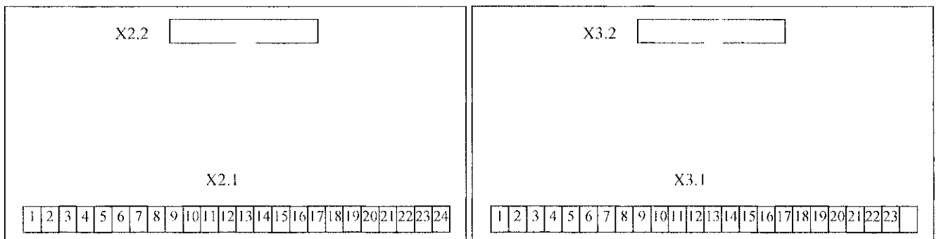
Рисунок А.2 - Силовая плата нижняя SP_POW(1)
