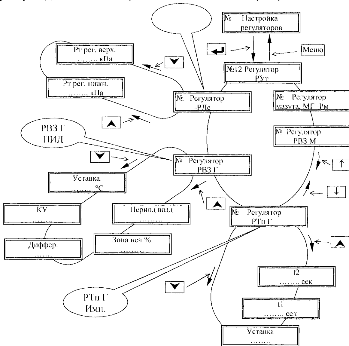
Рисунок 6.8 - Раздел основного меню наладчика «Настройка регуляторов»
