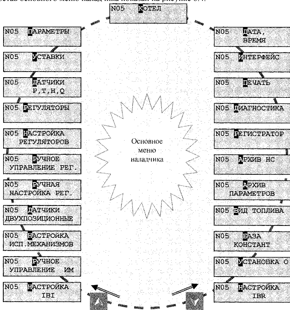
Рисунок 6.4 - Состав основного меню наладчика 6.6.2.1 Раздел основного меню наладчика «Уставки»
