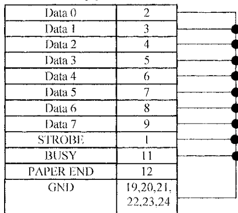
Интерфейс Centronics
