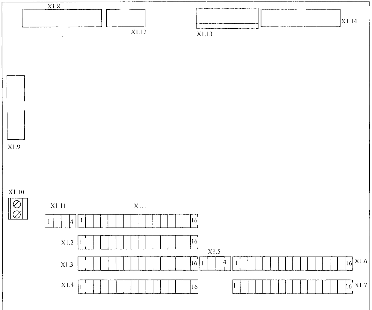
Рисунок А.1 - Расположение разъёмов на плате SP CPU и их нумерация.
