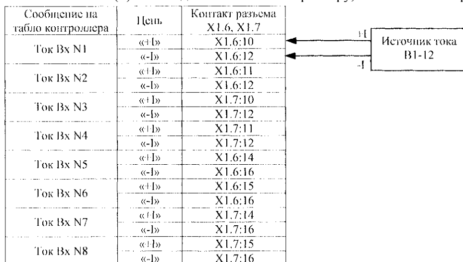
Рисунок Д.2 - Схема подключения источника тока при настройке IB1, при поверке токовых входов
