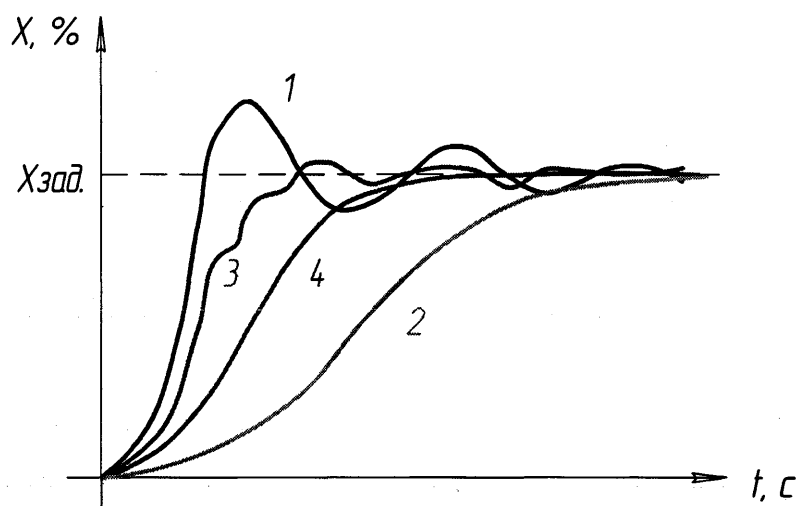
Рис.5 Графики переходных процессов
