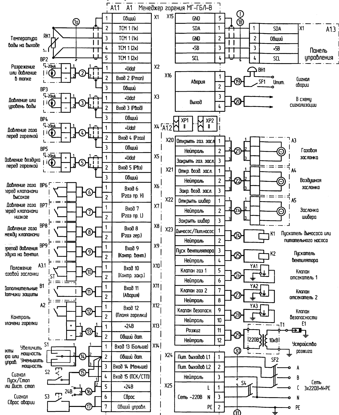
Рис.Г.1 Схема подключения модификации МГ-ГБЛ-В
