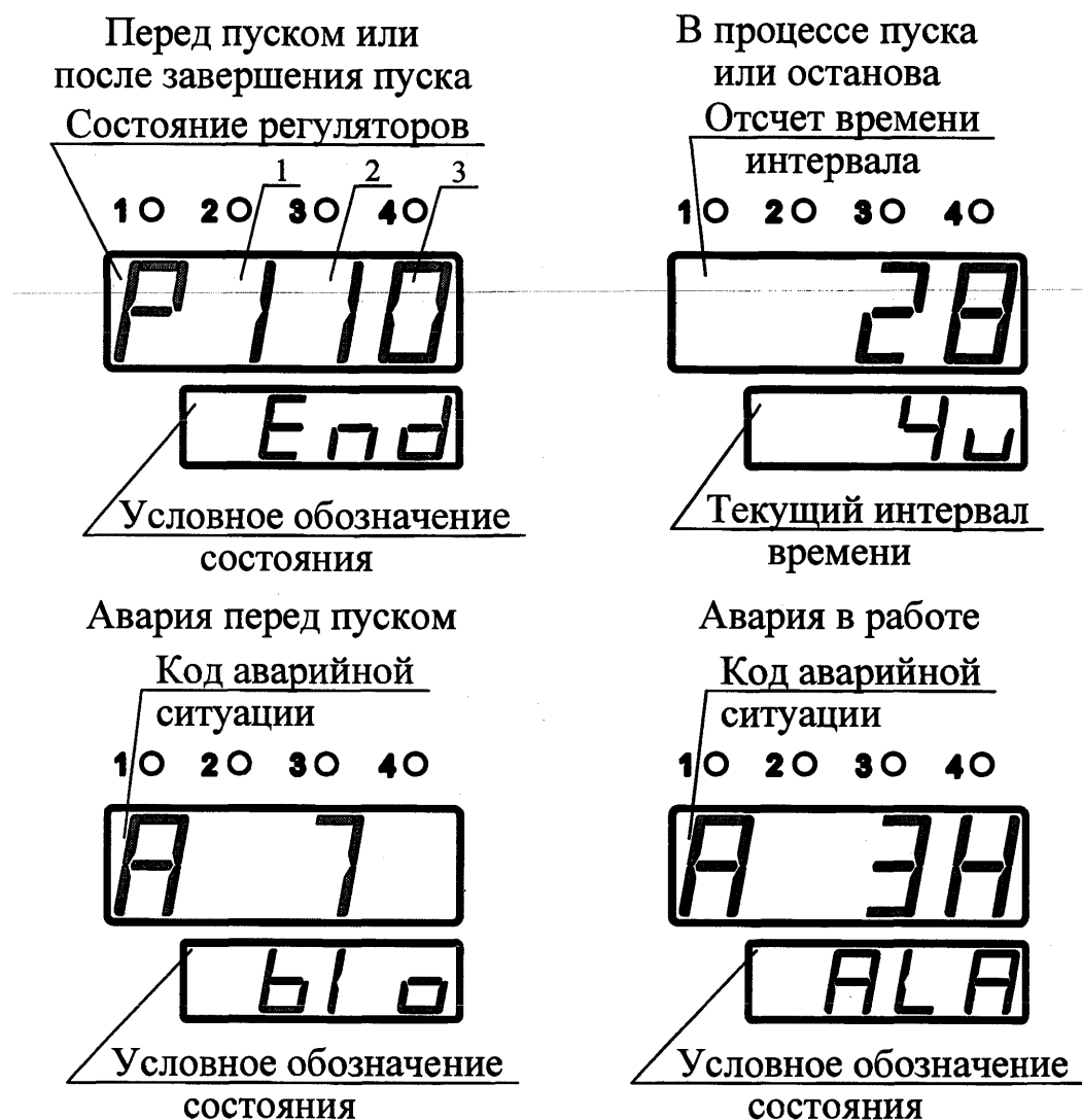
Рис.4 Индикация в дополнительном режиме отображения
