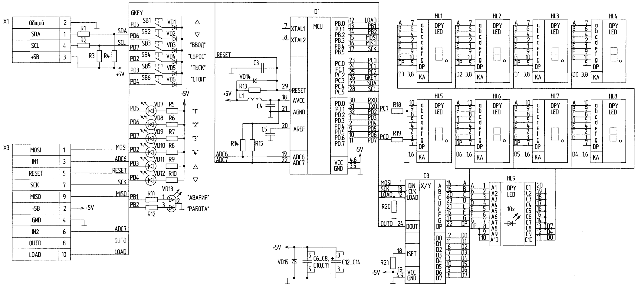
Рис. В.4 Схема электрическая принципиальная платы индикации
